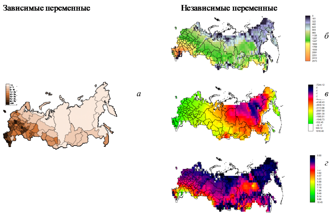
Рис. 1. Схема сопряженного анализа плотности населения (а) и климатических показателей: градусо-дней теплого периода (б); сумм отрицательных температур (в); индекса сухости (з)
